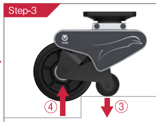
後輪が押し返される力を 前輪が路面を押し下す力に変換
